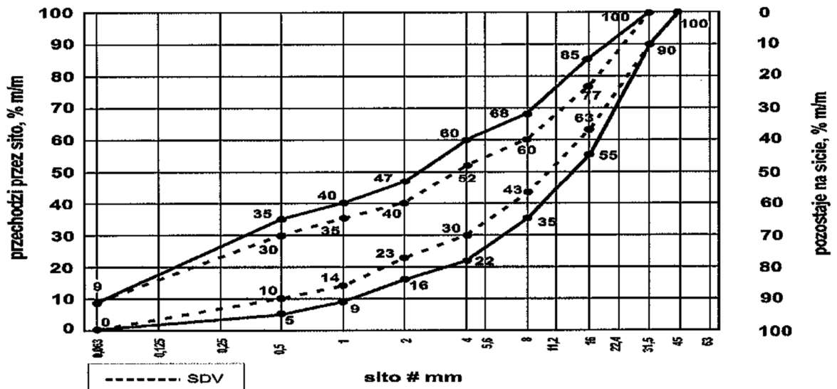
Rys. 2 Mieszanka kruszyw 0/31,5 do podbudowy zasadniczej pod chodnik, zjazd, pobocze
