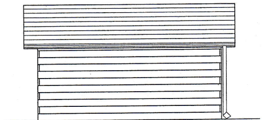
ELEWACJA TYLNA
