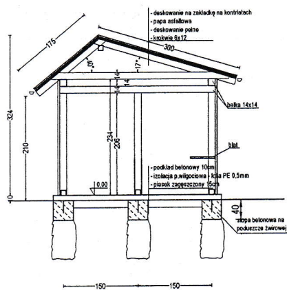
PRZEKRÓJ PIONOWY
