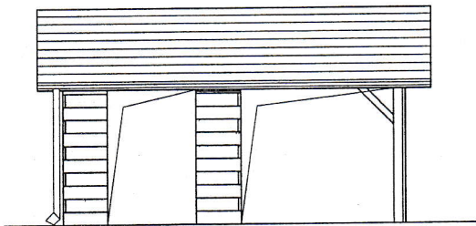
ELEWACJA FRONTOWA
