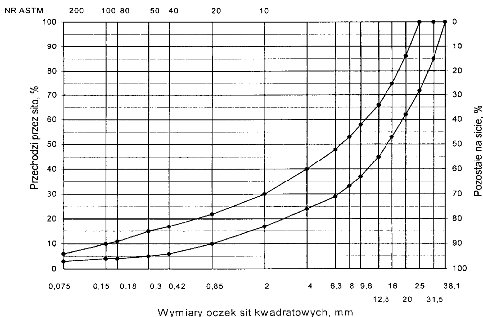
Rys. 1. Krzywe graniczne uziarnienia mieszanki mineralnej BA od 0 do 31,5 mm podbudowy
