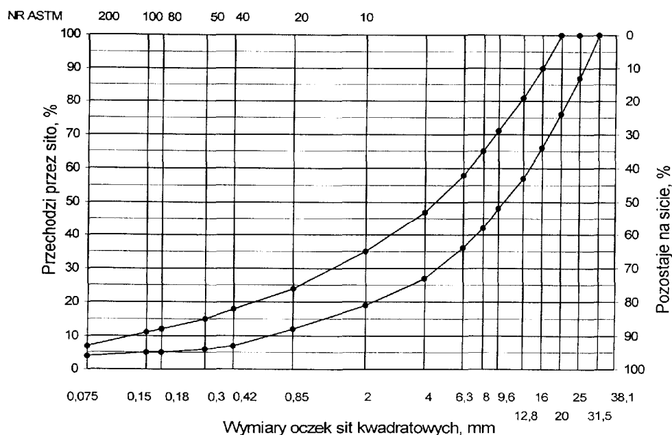
Rys.2. Krzywe graniczne uziarnienia mieszanki mineralnej BA od 0 do 25 mm podbudowy
