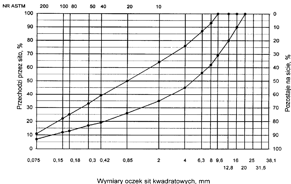
Rys. 1. Krzywe graniczne uziarnienia mieszanki mineralnej BA od 0 do 16mm, od 0 do 12,8 mm
